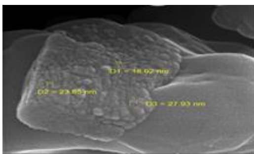
شکل ۲. تصویر SEM نانوذرات منگنز Figure 2. Nanomanganese SEM
