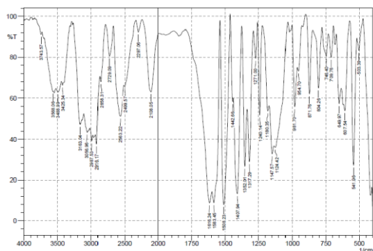
شکل ۱. تصویر FT-IR ذرات منگنزمتیونین Figure 1. Manganese methionine FT-I
