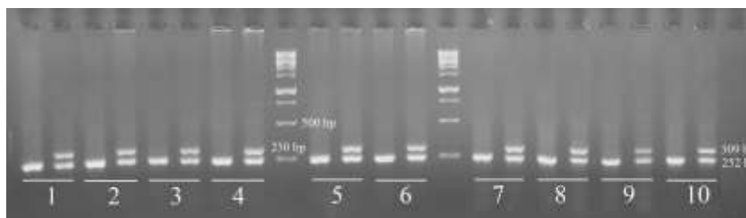
شکل ۵. نتایج ژل‌گذاری محصولات PCR به دست آمده از DNA استخراج شده از پر ده نژاد قناری ۱- آمیخته ۲- رسمی ۳- لانکشاير ۴- کرسست ۵- فری پارسیسی ۶- گلاستر فنسی ۷- اپال ۸- جیبیر ۹- موزائیک ۱۰- فیورینو Figure 5. Results of gelation of PCR products derived from DNA extracted from 10 Canary Canopy feathers. 1- Cross 2- Rasmi 3- Lancashire 4- Crest 5- Parisian Fril 6- Gloster Fancy 7- Opal 8- Jiber 9- Mosaik 10- Fiorino
