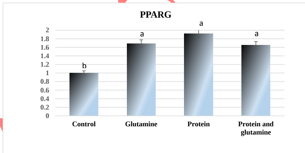
شکل ۳. تأثیر تیمارهای مختلف بر بیان نسبی ژن PPARG در عضله
