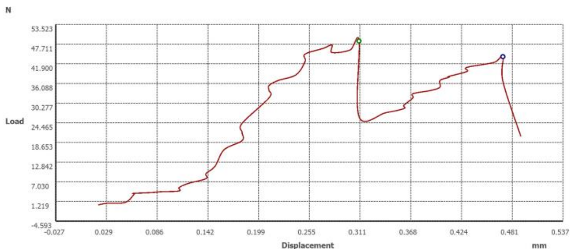
نمودار ۲. نقطه شکست استخوان ران در تیمار ۱۳ را نشان می دهد.
